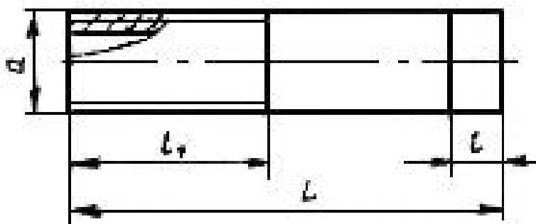
Чертеж. Основные размеры сгонов
